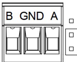
Résistance de terminaison désactivée
