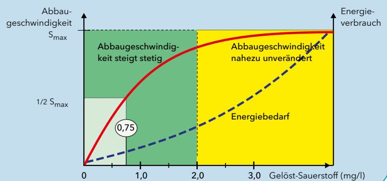
Abhängigkeit des \text{NH}_4 -N-Abbaus von der Sauerstoff-Konzentration
