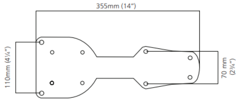
Manual Toilet Footprint
