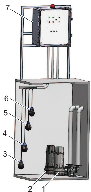
Figure 1: Installation typique du panneau de commande duplex 4NS
