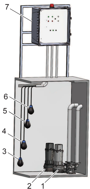
Figura 1: Instalación típica del panel de control dúplex 3SD/4SD
