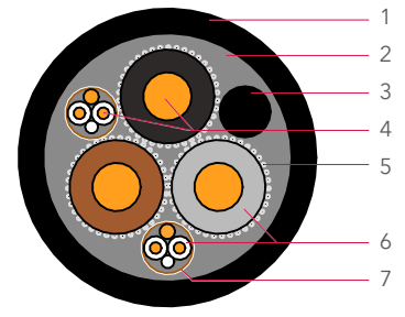
S3x70+3x25/3+S2(2x0.5) SUBCAB®
