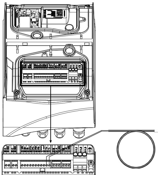
Figura 2: Diagrama de conexión para modelos trifásicos ecocirc XL
