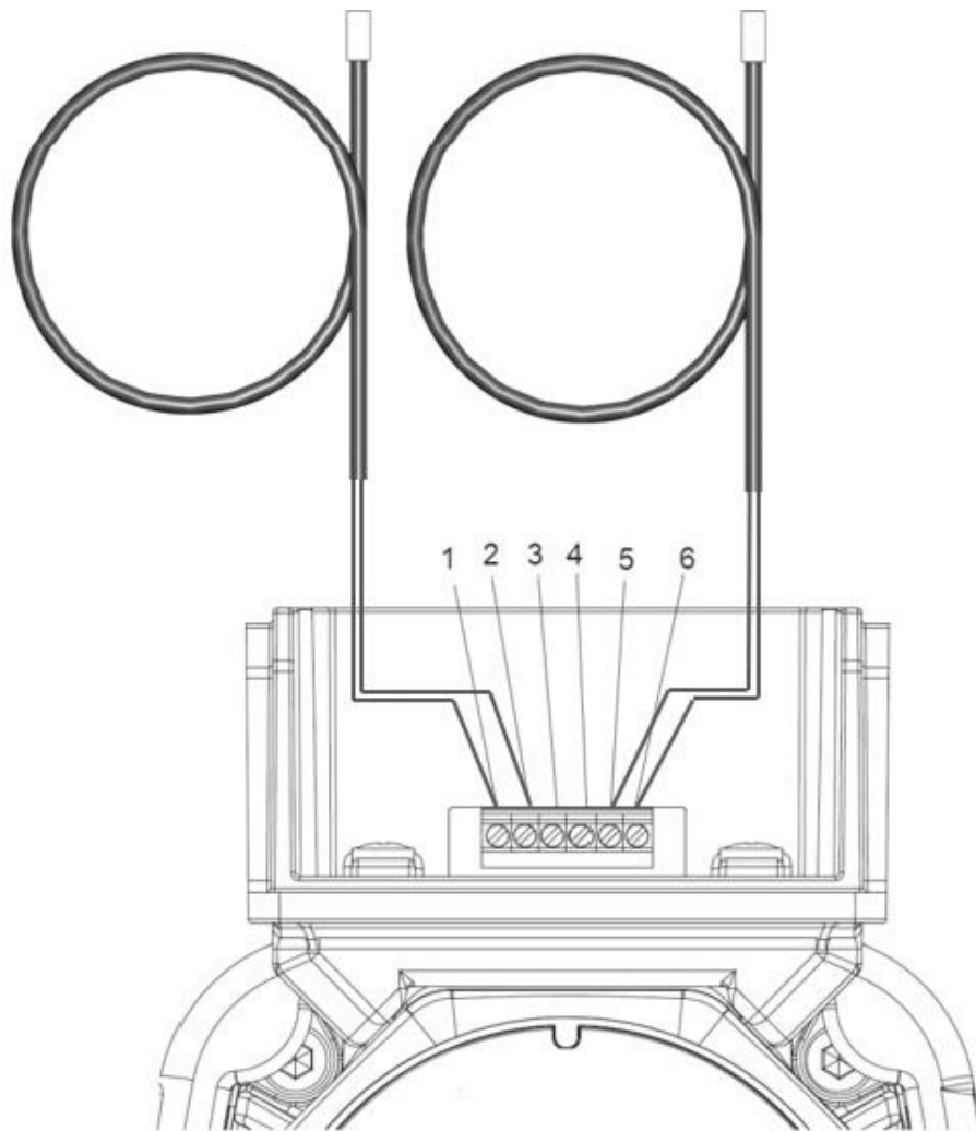
Figura 3: Diagrama de conexión para ecocirc 20-18+ para control de temperatura simple o delta T.
