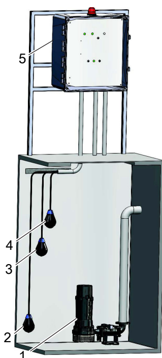
Figura 1: Instalación típica del panel de control simple 4DWC
